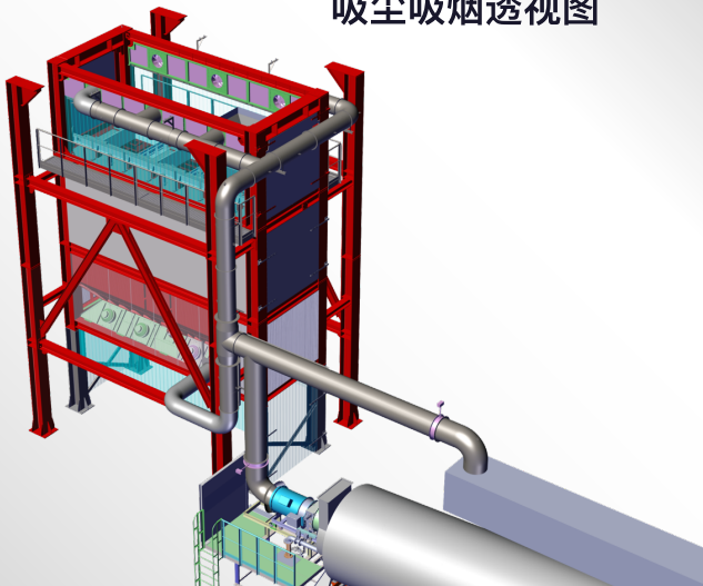
吸尘吸烟透视图
